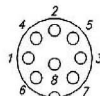
Anschluss BKS Ansicht von hinten auf den Stecker
