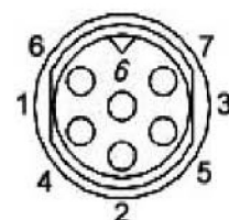
Gerätestecker (Ansicht Steckseite)
