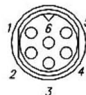
Gerätestecker (Ansicht Steckseite)
