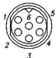
Gerätestecker (Ansicht Steckseite)
